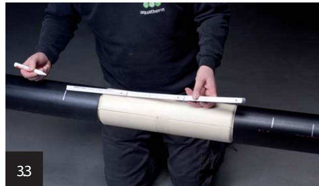
A zsugorkarmantyú helyének kijelölése
