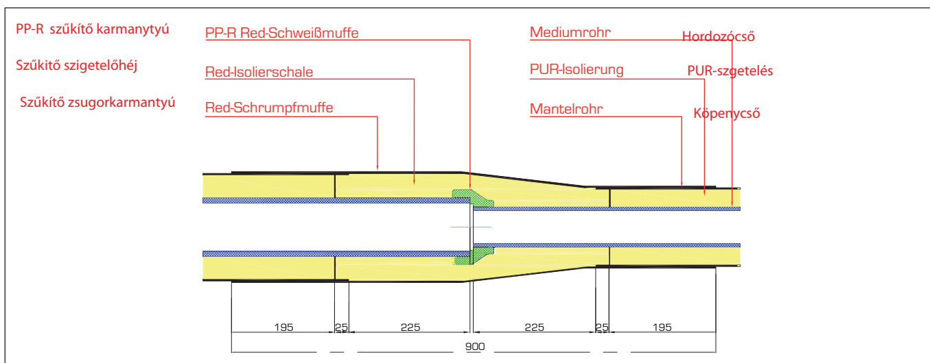
aquatherm ti-Szűkítő karmantyú
