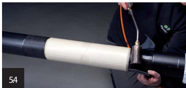
Az olvadó szalagok felhelyezése
